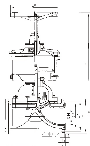
GG641Fx型气动隔膜阀(往复式)
