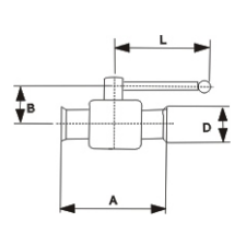
不锈钢卫生级直通式球阀
