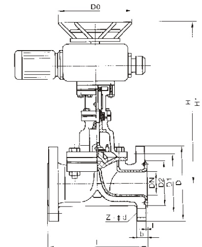
GG941Fx电动隔膜阀(堰式)
