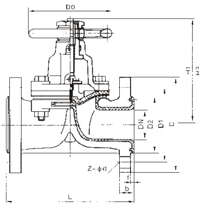
GG41Fx型手动隔膜阀(堰式)
