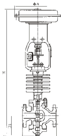
(ZMBN 散热型) (ZMBN heat radiation type)
